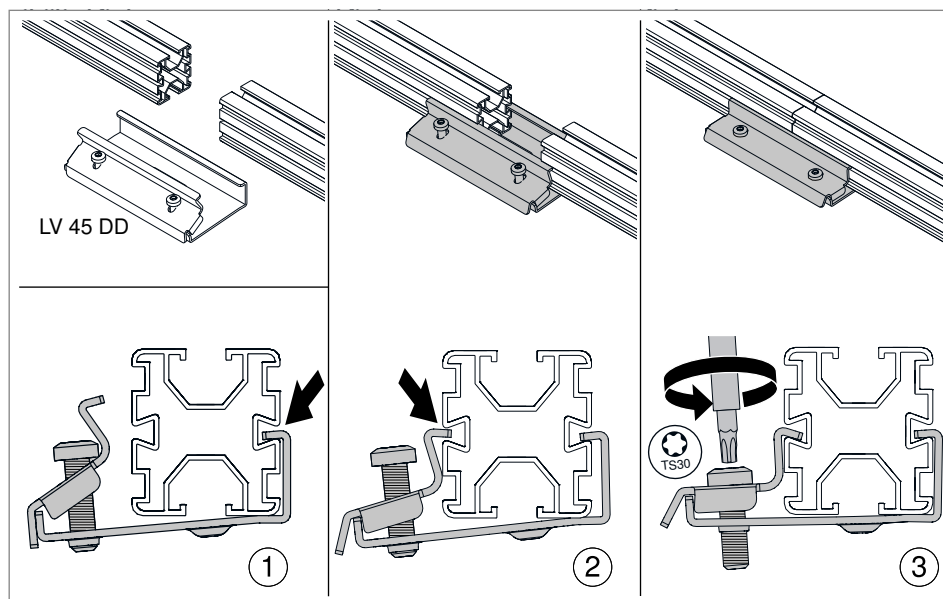
Rys. 35: Montaż łączników wzdłużnych
