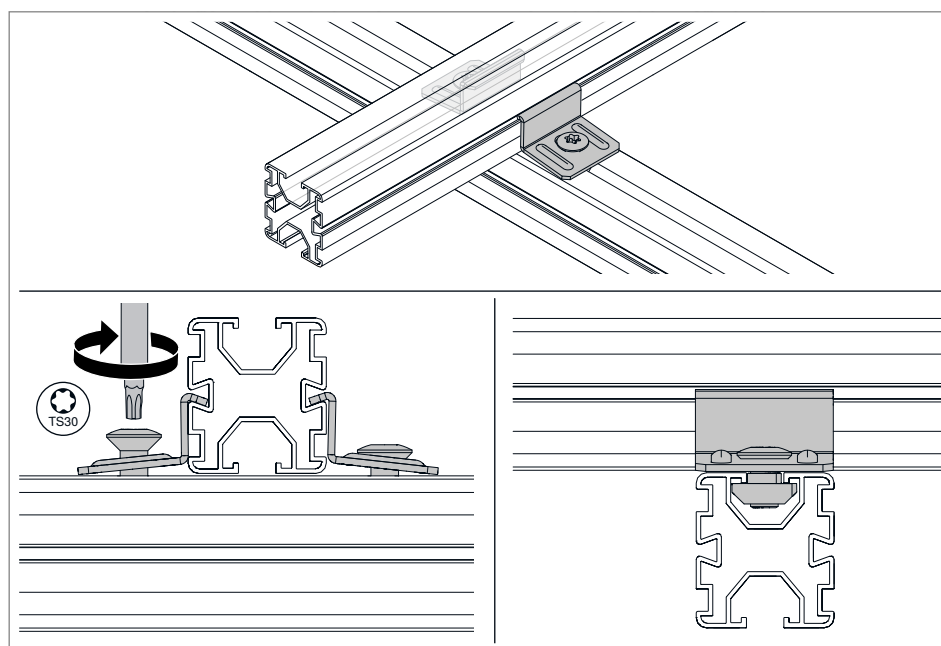
Rys. 37: Przykręcanie łącznika krzyżowego
