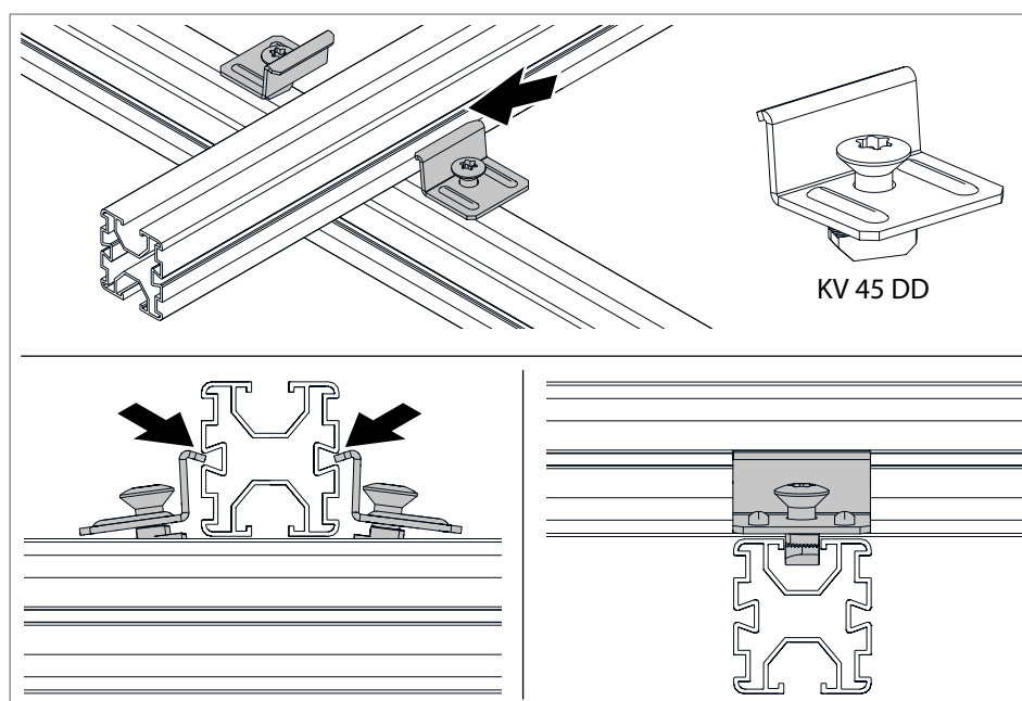
Rys. 36: Umieszczanie łącznika krzyżowego
